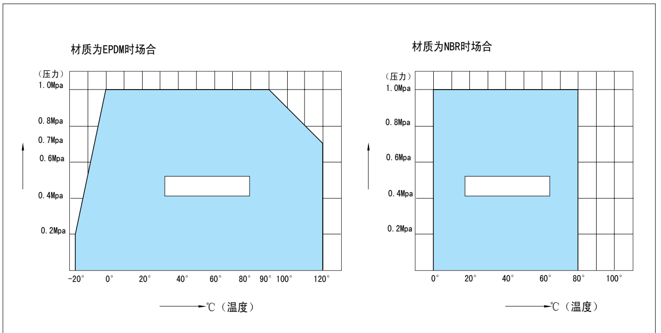
700G 压力-温度等级
